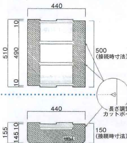
510×440×1~7(スロープ形状)
